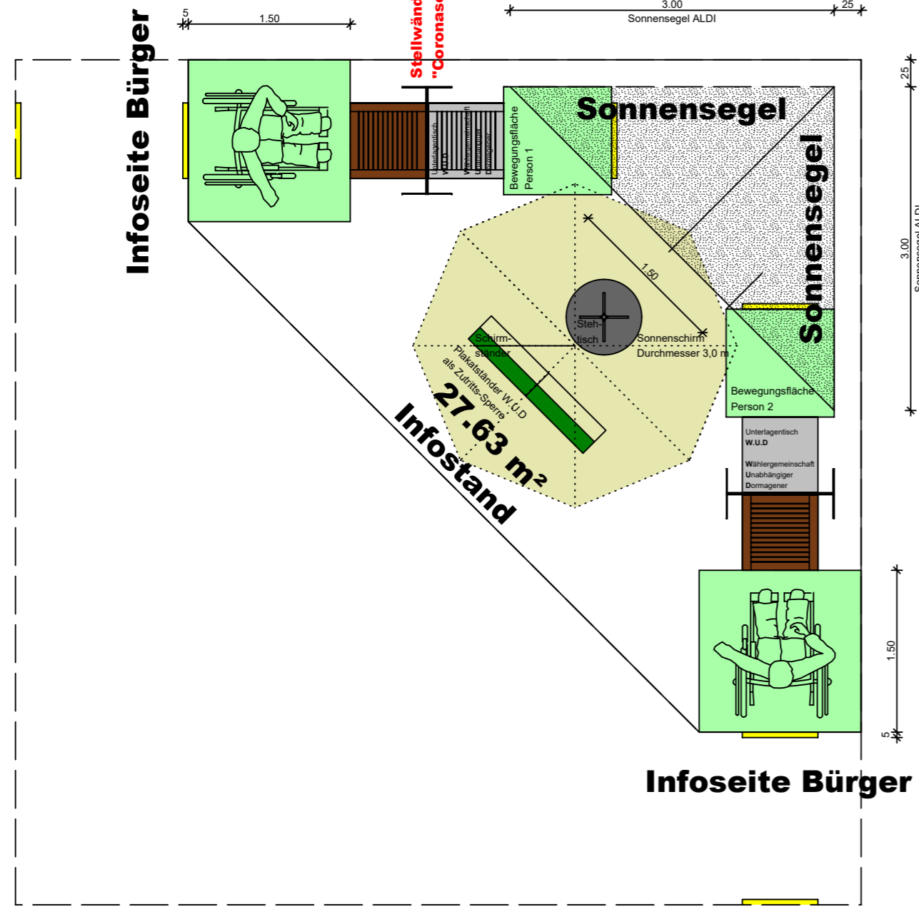
Grundriss M 1:50
